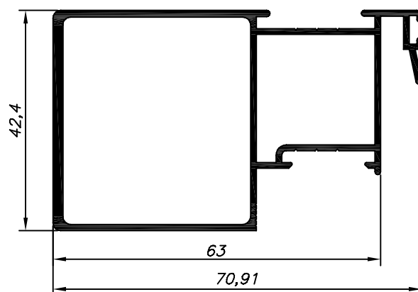
SU-049 4,500 Kg/Barra 4,6m Escovinha Base 5
