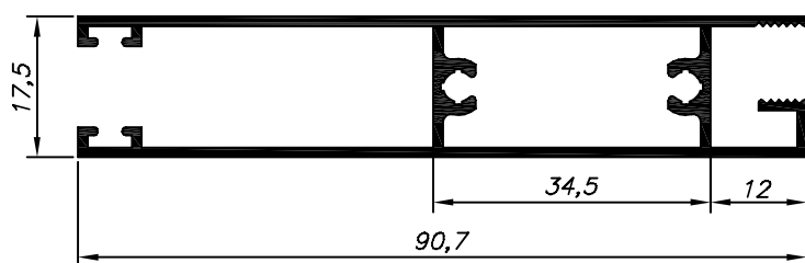
MP-354 5.820 Kg/Barra 6m Escovinha Base 5
