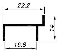
DS-036 0,770 Kg/Barra 6m
