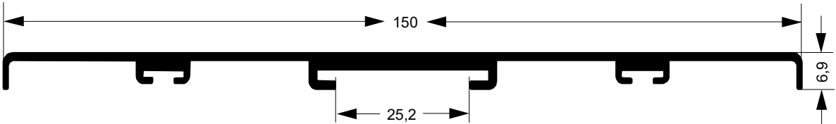
DES - 005 6,659kg/Barra 6m
