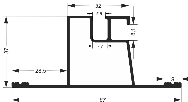
POL-039 5.788kg/6m
