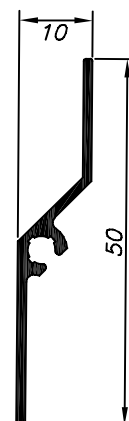
DV-113 1.500 Kg/Barra 6m
