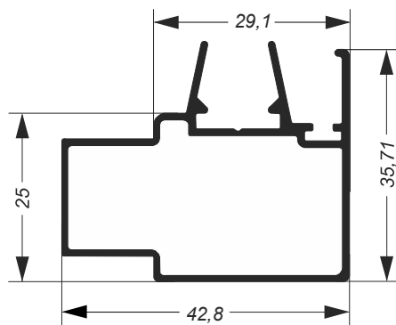
SU-038 3,471 Kg/Barra 6m Escovinha Base 5
