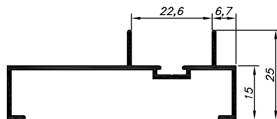
MP-360 2.250 Kg/Barra 6m
