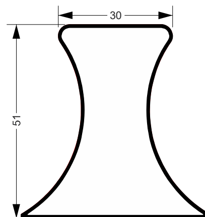
3.100 Kg/Barra 6m
