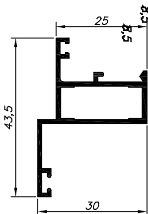
25-005 2.500 Kg/Barra 6m Escovinha Base 5
