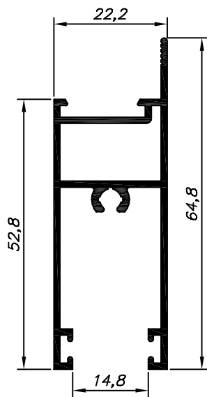
SU-246 3,750 Kg/Barra 6m Escovinha Base 5
