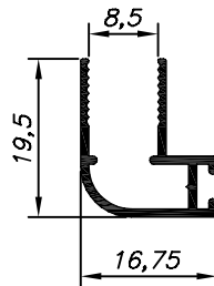
BX-271 1,040 Kg/Barra 6m Escovinha Base 5
