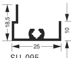
SU-095 1.439 Kg/Barra 6m
