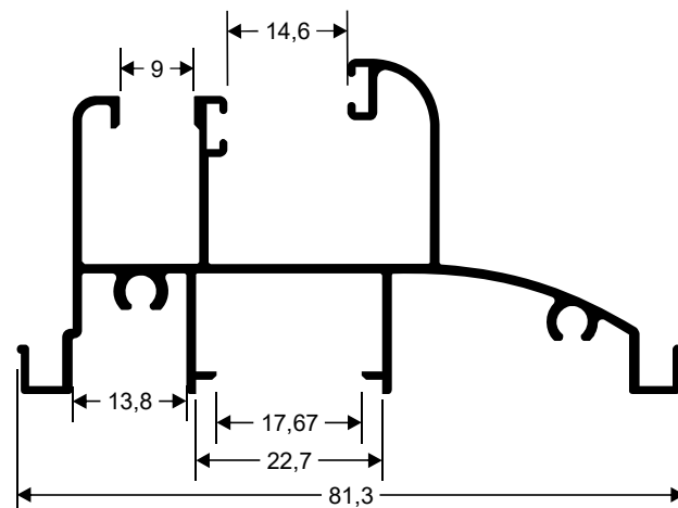
JV-002 4.878 kg/Barra 6m
