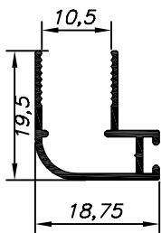
BX-251 1,080 Kg/Barra 6m Escovinha Base 5
