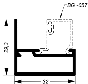
NOE - 086 2,389 Kg/Barra 6m
