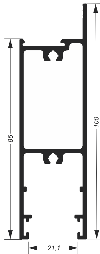
NOE-007 7,728Kg/Barra 6m Escovinha Base 7,5
