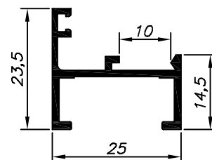
25-027 1.600 Kg/Barra 6m Escovinha Base 5
