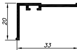
CL-015 1.300 Kg/Barra 6m Escovinha Base 5
