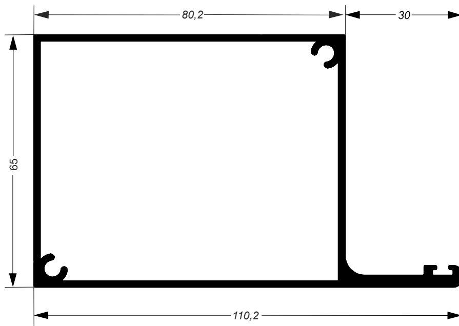
MCP -005 10.481Kg/Barra 6m
