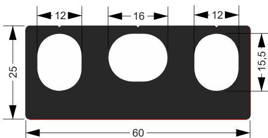
01.0181 18.190 Kg/Barra 6m
