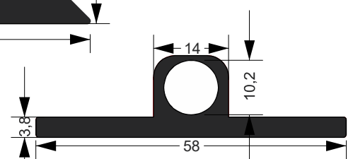
01.0180 5.227 Kg/Barra 6m
