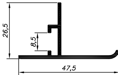
LM-101 2.080 Kg/Barra 6m
