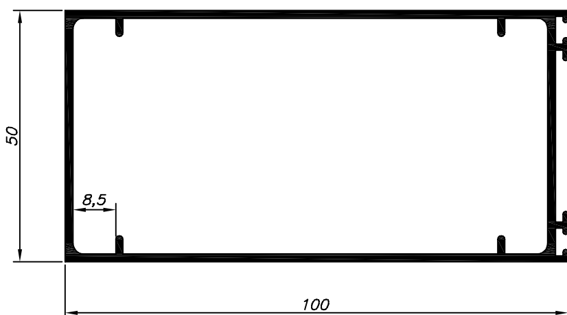
MEG-002 8,969 Kg/Barra 6m Borracha GUA008
