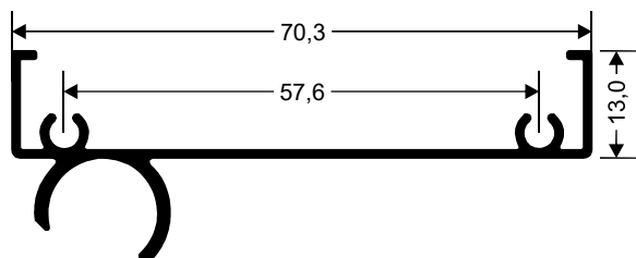
GNS-006 2.660 Kg/Barra 6m
