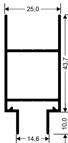
SU-191 3,102 Kg/Barra 6m
