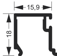
NOE-059 1.128Kg/Barra 6m
