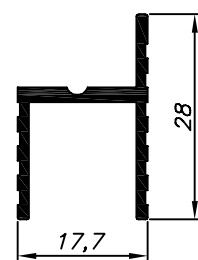
BX-106 1.458 Kg/Barra 6m
