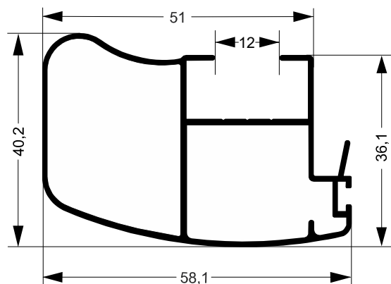
SU-028 4.785 Kg/Barra 6m Escovinha Base 5
