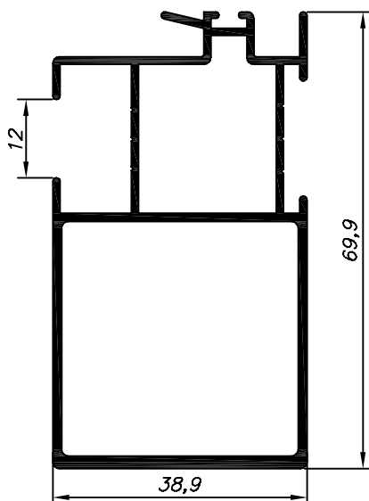
SU-061 4,513 Kg/Barra 4,6m Escovinha Base 5
