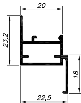
20-049 1.800 Kg/Barra 6m
