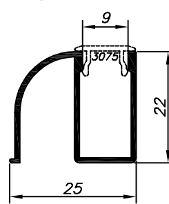
BX-059 1,530 Kg/Barra 6m Escovinha Base 5
