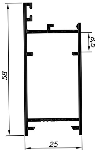
25-542 3.760 Kg/Barra 6m Escovinha Base 5
