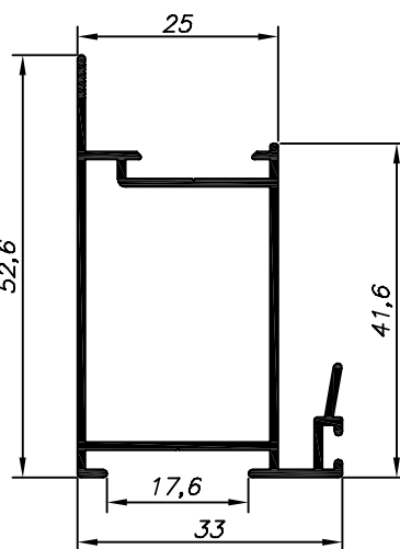
SU-283 2,560 Kg/Barra 4,6m Escovinha Base 5
