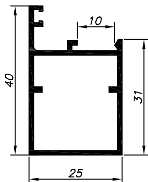
25-016 2.600 Kg/Barra 6m Escovinha Base 5
