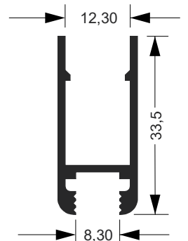
KP-004 2.224 Kg/Barra 6m
