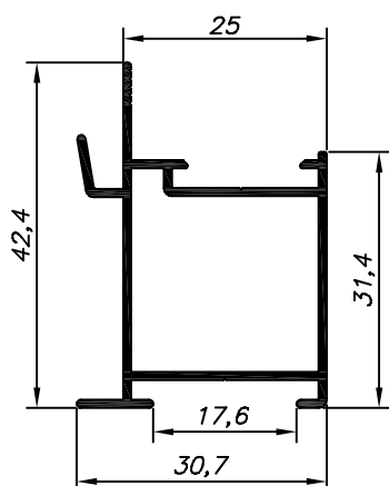
SU-040 2,610 Kg/Barra 6m 2,020 Kg/Barra 4,6m Escovinha Base 5
