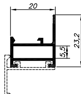
20-051 1.400 Kg/Barra 6m
