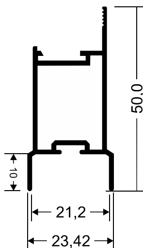
MP-318 2.700 kg/Barra 6m
