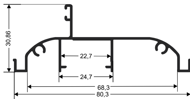
JM-001 3.465 Kg/Barra 6m
