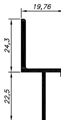
20-142 1.850 Kg/Barra 6m
