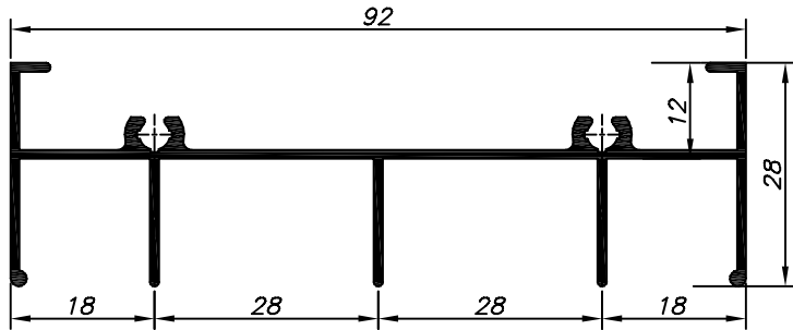
MP-366 4.540 Kg/Barra 6m
