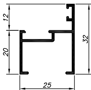
25-311 1.830 Kg/Barra 6m
