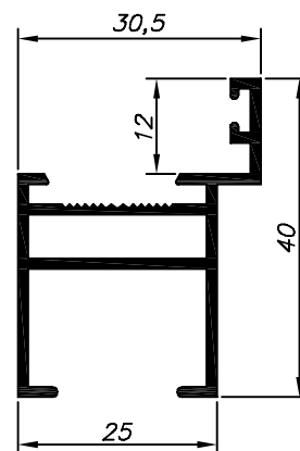
25-540 3.240 Kg/Barra 6m Escovinha Base 5
