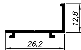
SU-084 0,800 Kg/Barra 6m
