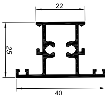
25-026 3.050 Kg/Barra 6m
