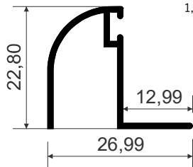
SP-001 1,419Kg/Barra 6m Escovinha Base 5
