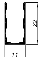
BX-103 0,840 Kg/Barra 6m
