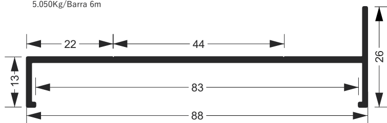
SUP-2648 3.022Kg/Barra 6m
