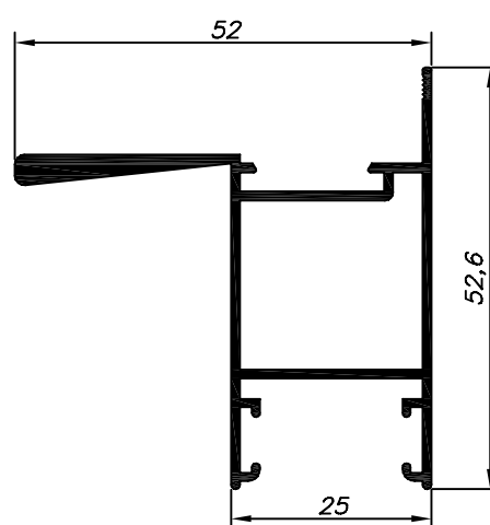
SU-250 4,830 Kg/Barra 6m 3,703 Kg/Barra 4,6m Escovinha Base 7,5
