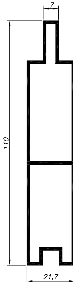
LB-070 6.820 Kg/Barra 6m
