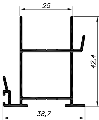
SU-069 3,150 Kg/Barra 6m 2,420 Kg/Barra 4,6m Escovinha Base 5
