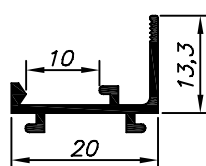
20-053 0,900 Kg/Barra 6m
