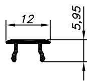
3075 0,330 Kg/Barra 6m
