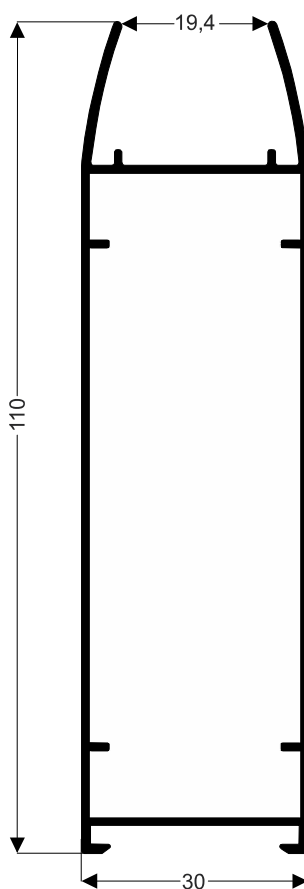
EMX-004 5,951Kg/Barra 6m
