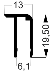
DES-883 1,014Kg/Barra 6m ESPESSURA = 1.2mm
