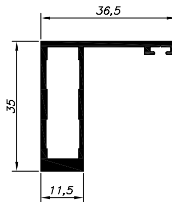
PS-002 3.230 Kg/Barra 6m Borracha GUAPS01
