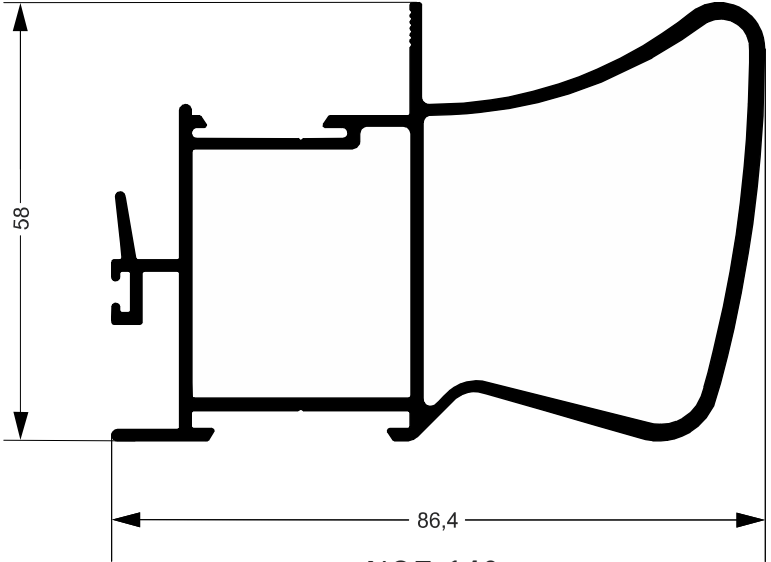
NOE-140 9,941Kg/Barra 6m Escovinha Base 5
