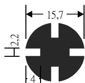
LM-103 2.640kg/Barra 6m
