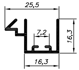
DS-1391 1,310 Kg/Barra 6m Escovinha Base 5
