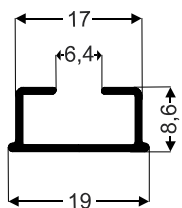
TRI-041 0,581Kg/Barra 6m
