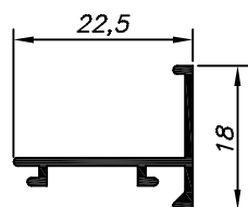
20-055 0,930 Kg/Barra 6m
