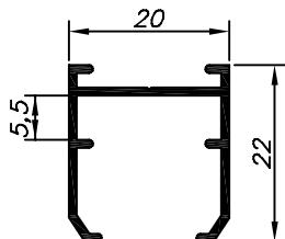
20-050 1.500 Kg/Barra 6m
