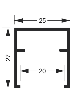
SU-093 1,848 Kg/Barra 6m
