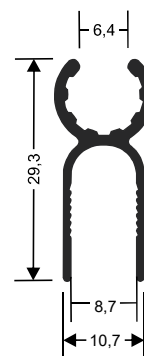
JM-004 1.412 Kg/Barra 6m
