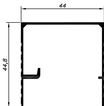
SUPRA-109 2.800 Kg/Barra 6m
