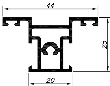
MM-376 3.126 Kg/Barra 6m
