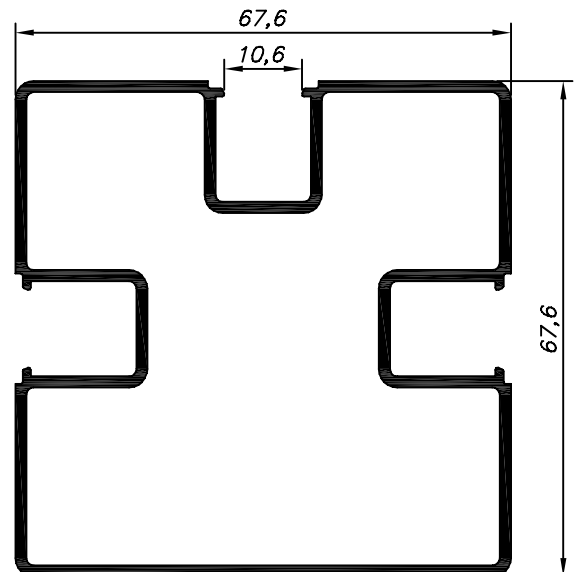
GR-017 9.220 Kg/Barra 6m
