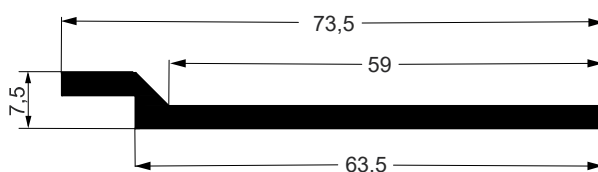
11.0035 4.111Kg/Barra 3m
