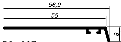
PS-007 1.422 Kg/Barra 6m Borracha GUA007
