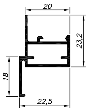
20-048 1.800 Kg/Barra 6m
