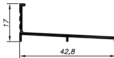
BX-153 1.164 Kg/Barra 6m
