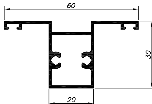
25-023 3.400 Kg/Barra 6m
