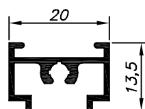
20-054 1.250 Kg/Barra 6m
