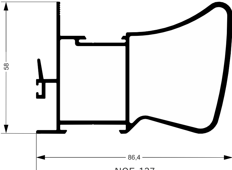
NOE-137 9,941Kg/Barra 6m Escovinha Base 5
