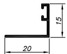
BX-005 0,812 Kg/Barra 6m Escovinha Base 5
