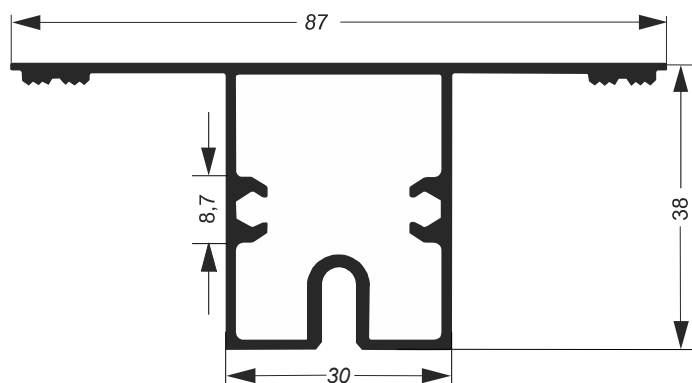
POL-033 6.448kg/6m
