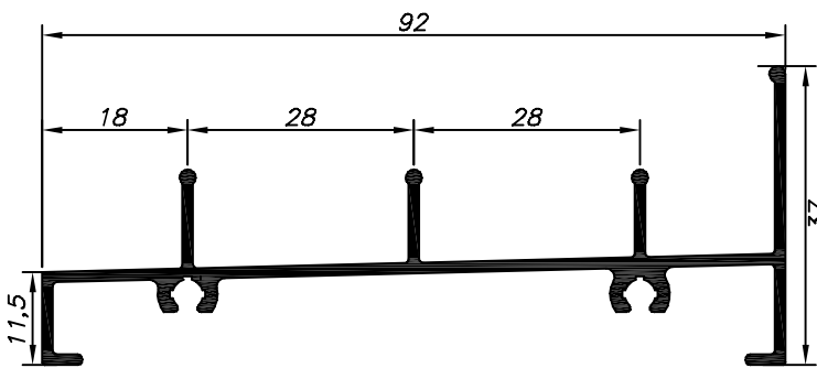
MP-367 4.900 Kg/Barra 6m
