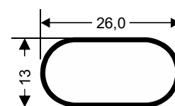
TG-076 0.865 Kg/Barra 6m
