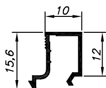
BG-035 0,730 Kg/Barra 6m
