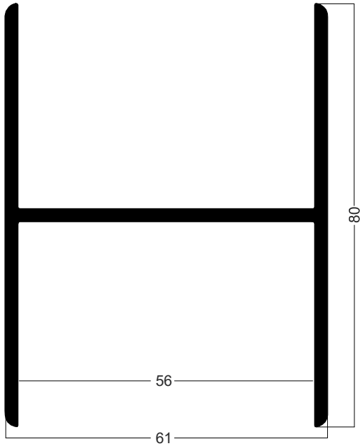
SMX-027 8,955Kg/Barra 6m
