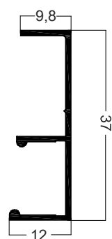
MP-347 1.150Kg/Barra 6m
