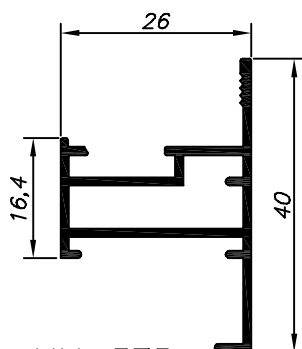
MM-375 2.340 Kg/Barra 6m
