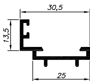
25-548 1.700 Kg/Barra 6m Escovinha Base 5
