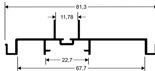
JV-003 2.808 kg/Barra 6m
