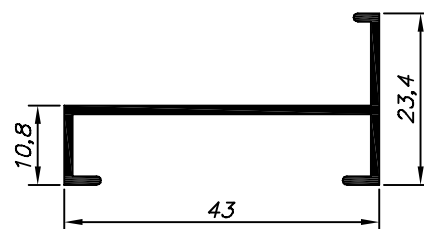
25-513 1.650 Kg/Barra 6m
