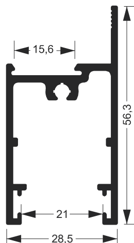
NOE-006 4.270Kg/Barra 6m Escovinha Base 7,5
