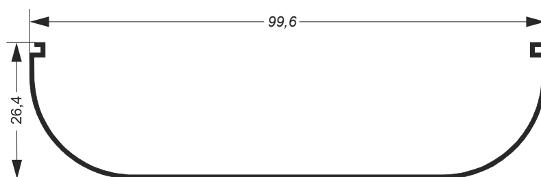
DS-202B 2.013Kg/Barra 6m
