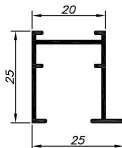
20-103 1.450 Kg/Barra 6m
