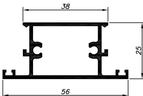
25-508 4.100 Kg/Barra 6m
