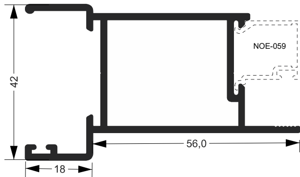
NOE-051 5,554Kg/Barra 6m Escovinha Base 5
