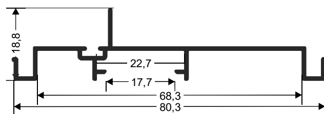
JM-003 2.514 Kg/Barra 6m
