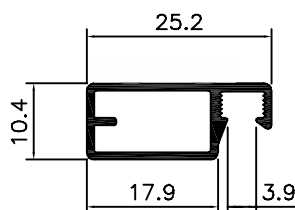
25-551 1.188 Kg/Barra 6m
