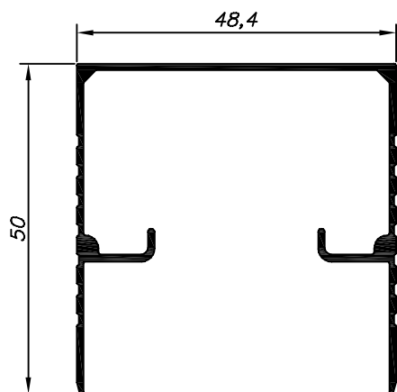
BX-109 3.140 Kg/Barra 6m
