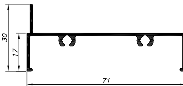
SU-004 3.000 Kg/Barra 6m
