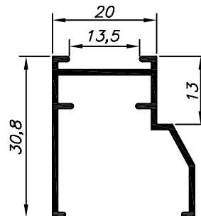
20-212 1.600 Kg/Barra 6m
