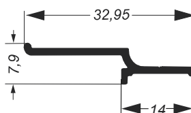
SUP-2653 0.910Kg/Barra 6m
