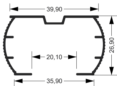
DES-017 1,775 Kg/Barra 6m
