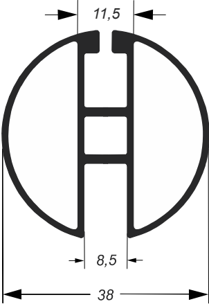
HAN-001 4,474Kg/Barra 6m
