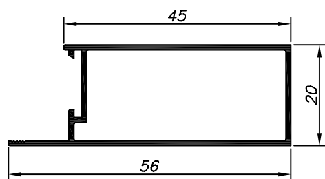
MP-336 1.800 Kg/Barra 4,6m
