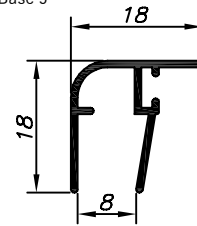
BX-093 0,910 Kg/Barra 6m Escovinha Base 5
