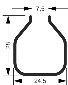
DES-013 1,676 Kg/Barra 6m
