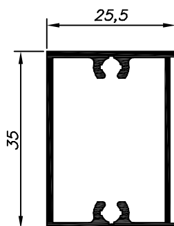
CG - 012 3.100 Kg/Barra 6m
