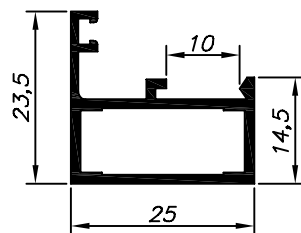
25-001 1.920 Kg/Barra 6m Escovinha Base 5
