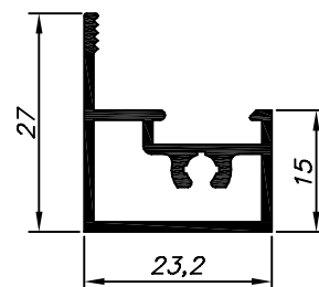
25-301 2.100 Kg/Barra 6m
