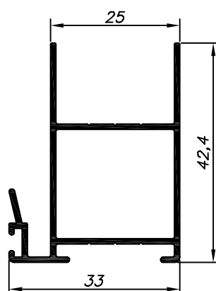
SU-070 2,850 Kg/Barra 6m 2,190 Kg/Barra 4,6m Escovinha Base 5
