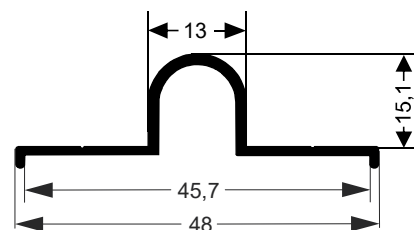
1.577Kg/Barra 6m Parafusado
