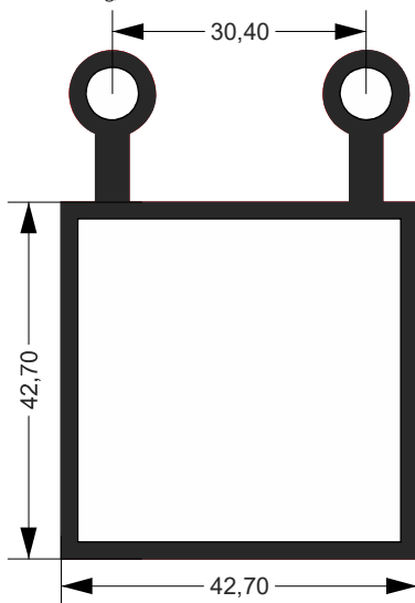
DS-001 8.800 Kg/Barra 6m
