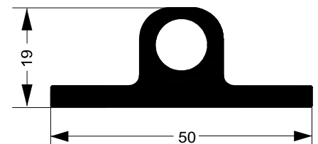
11.0013 6.151 Kg/Barra 6m
