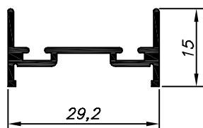
25-021 1.500 Kg/Barra 6m
