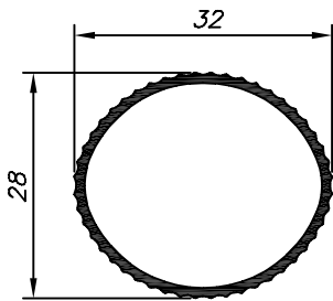
ALU-001 1.770 Kg/Barra 6m
