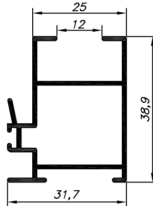
SU-056 3,000 Kg/Barra 6m 2,190 Kg/Barra 4,6m Escovinha Base 5
