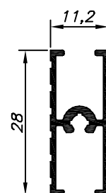
SUPRA-105 1.270 Kg/Barra 6m
