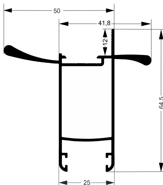
GNS-052 5.854 Kg/Barra 6m Escovinha Base 5
