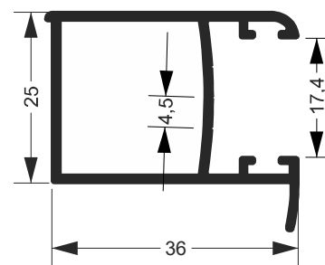
SUP-2649 2.944Kg/Barra 6m
