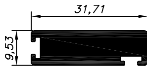
01.0155 4.600 Kg/Barra 6m
