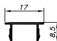
3074 0,530 Kg/Barra 6m
