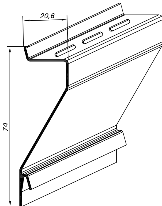
US-285 1.780 Kg/Barra 6m
