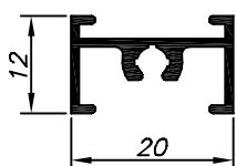
20-052 1.160 Kg/Barra 6m
