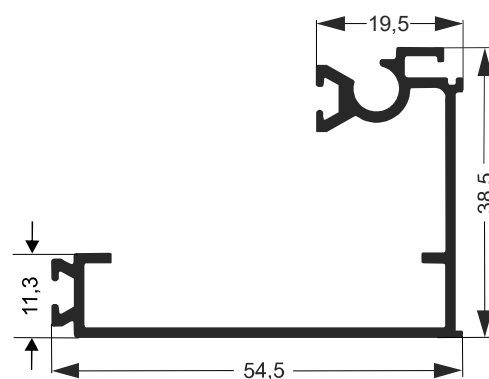
POL-030 3.900Kg/Barra 6m
