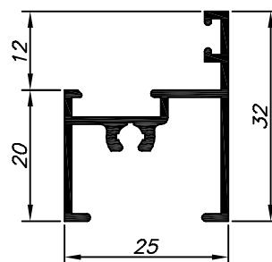
25-312 2.100 Kg/Barra 6m Escovinha Base 5
