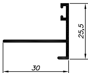
25-677 1.300 Kg/Barra 6m Escovinha Base 5
