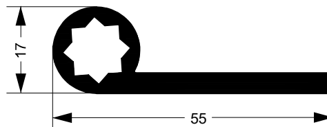
11.0084 5.075 Kg/Barra 6m
