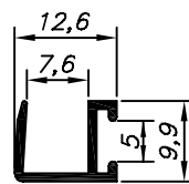
BX-126 0,560 Kg/Barra 6m Escovinha Base 7
