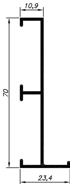
25-514 2.430 Kg/Barra 6m
