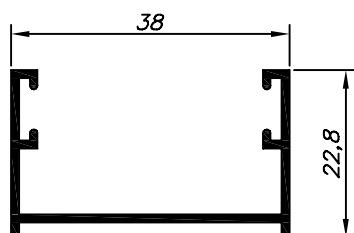
ME-024 2.060Kg/Barra 6m Escovinha Base 7
