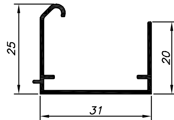
LM-102 1.570 Kg/Barra 6m
