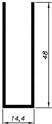
PU-048 2,700 kg/Barra 6m
