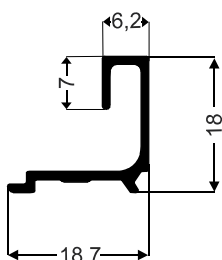
NOE-027 0,878Kg/Barra 6m
