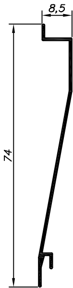
VZ-024 1.410 Kg/Barra 6m
