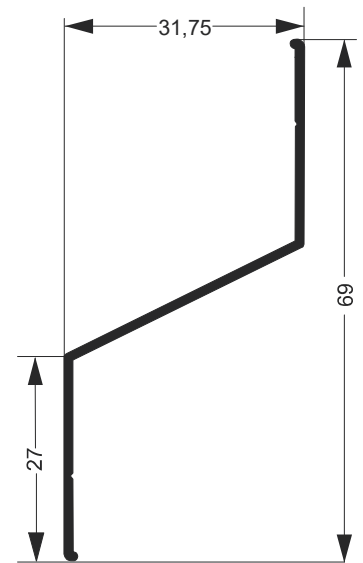
DEL-090 1.848Kg/Barra 6m
