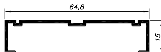
MP-397 2.280 Kg/Barra 6m
