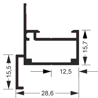
SU-097 2.462 Kg/Barra 6m
