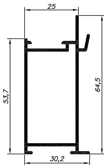
SU-243 3,060 Kg/Barra 4,6m
