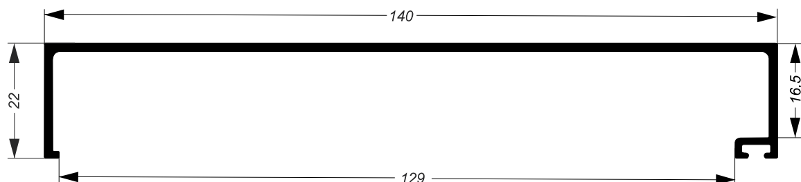
NOE-170 5.451Kg/Barra 6m
