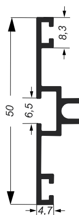
MEG-003 2.877kg/Barra 6m Borracha GUA008
