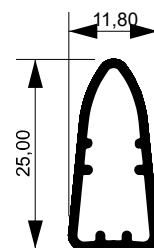
DES-019 1,131Kg/Barra 6m
