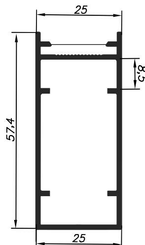
25-543 3.900 Kg/Barra 6m
